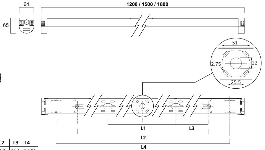
START Batten 1200 /1500 /1800
